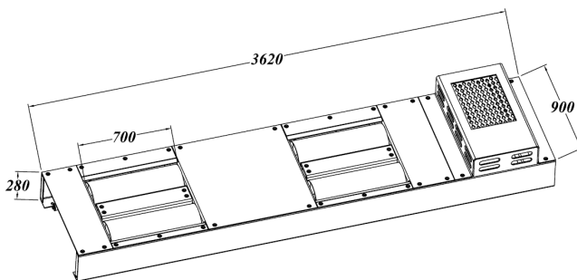
Mechanika méretei
