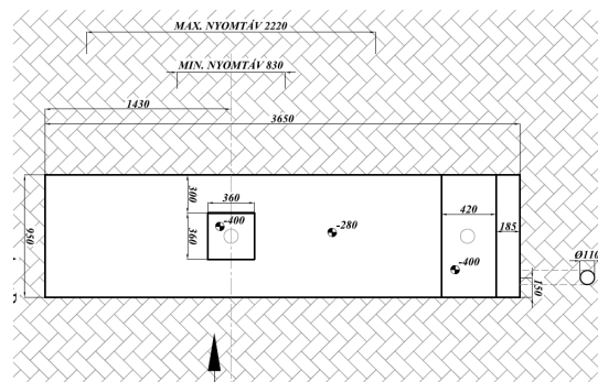
Telepítési vázlat
