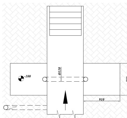
Telepítési vázlat
